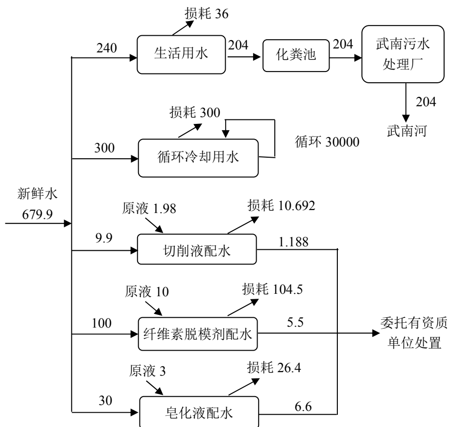
图 2-1 本项目水平衡图 (t/a)
