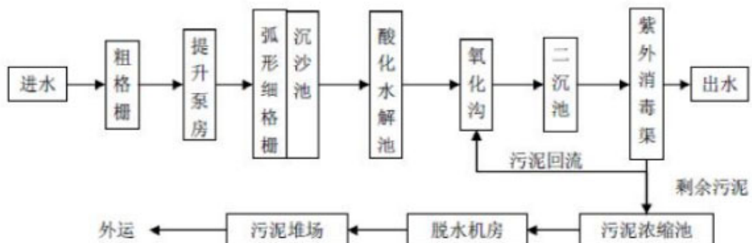
图 4-2 武南污水处理厂废水处理工艺流程图
